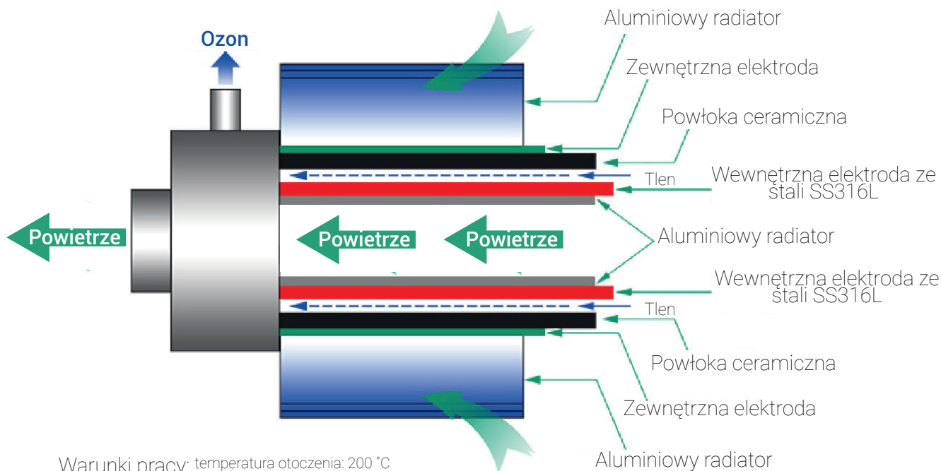
Budowa ogniwa
