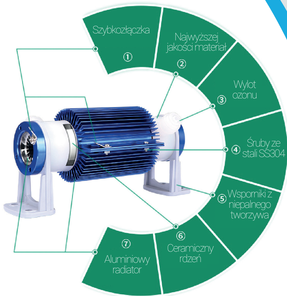
Budowa ogniwa
